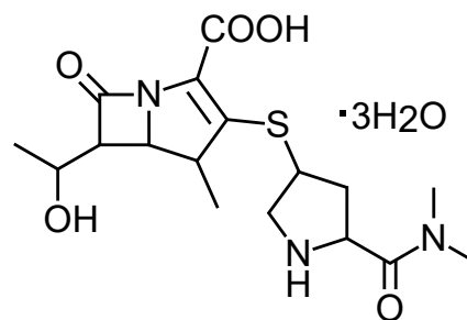
meropenem trihydrate [M+H] + m/z 384.1
