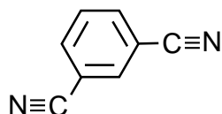
isophthalonitrile ( m -)
