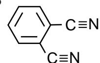
phthalonitrile ( o -)
