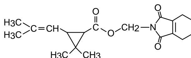
phthalthrin (tetramethrin)
